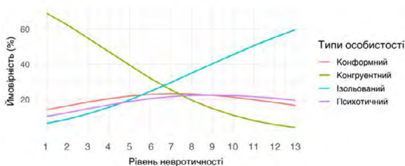
Рис. 2. Проста модель мультиномінальної логістичної регресії
